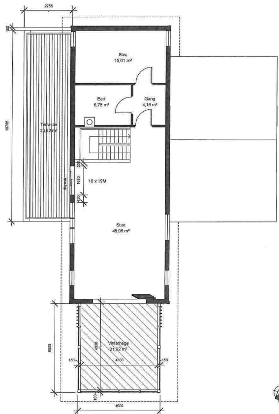
PLAN 2. ETASJE
