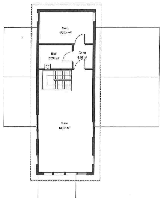
Plan 2.etasje
