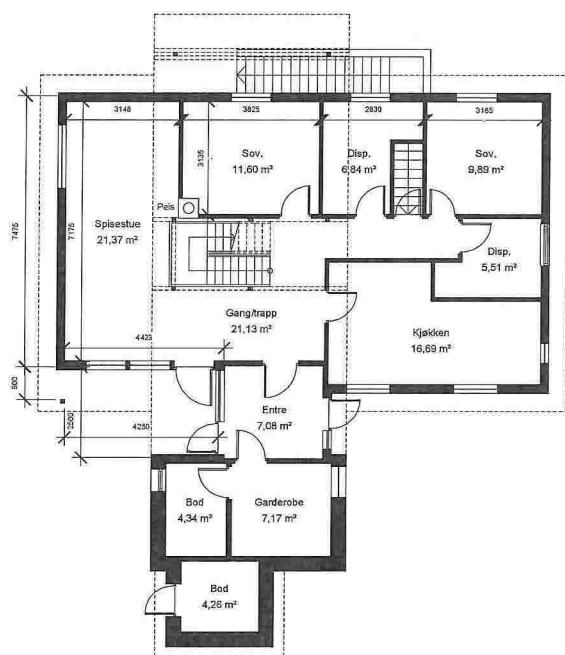
Plan 1.etasje
