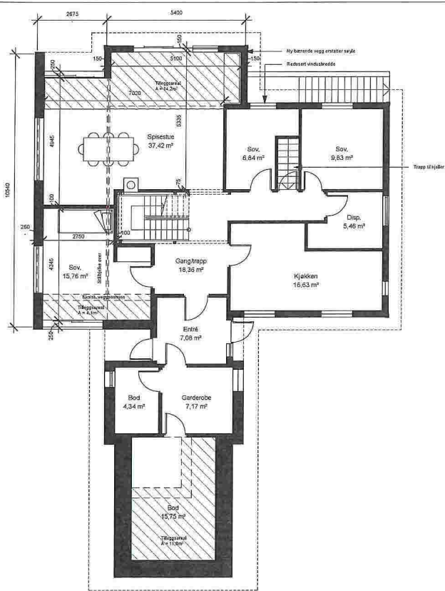
PLAN 1. ETASJE
