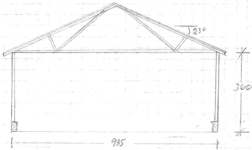
SNITT NORD BYGG UNDER REHALITERING
