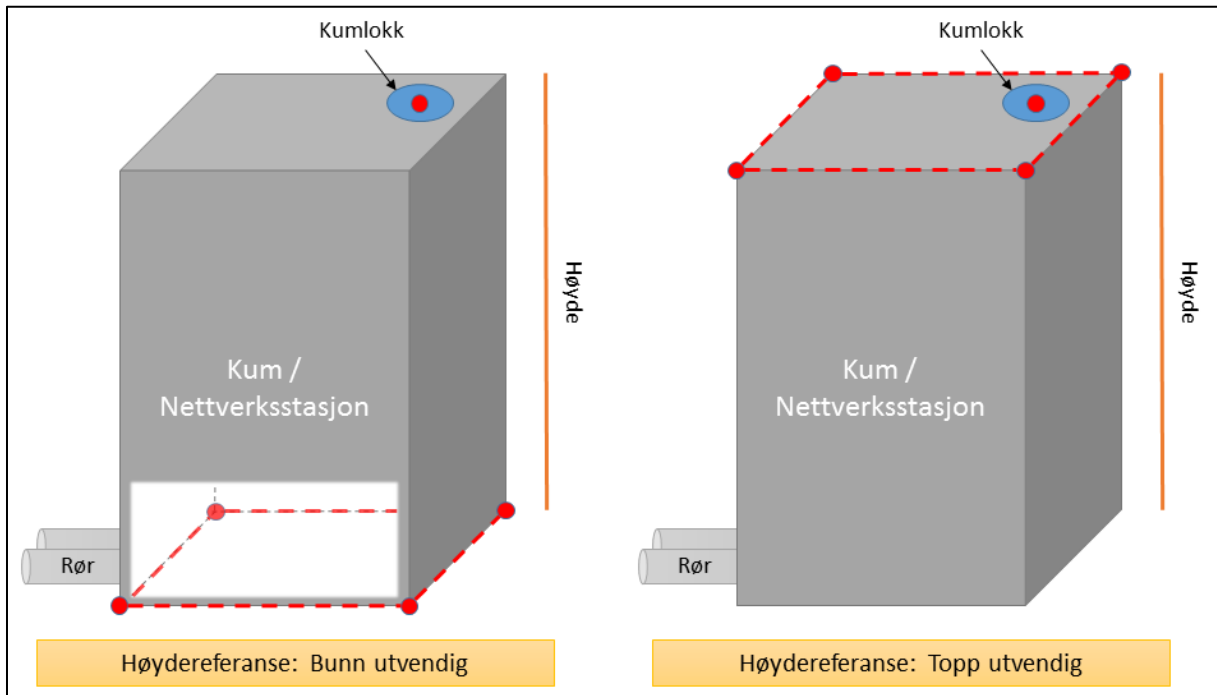
Figur 22: Alle ikke sirkulære kplingsobjekt skal registreres med hjørnekoordinater, primært bunn (alternativt topp), og høyde angivelse. Kplingsobjektets adkomst, her illustrert i form av kumlokk, skal stedfestes med senterpunkt for adkomsten.
