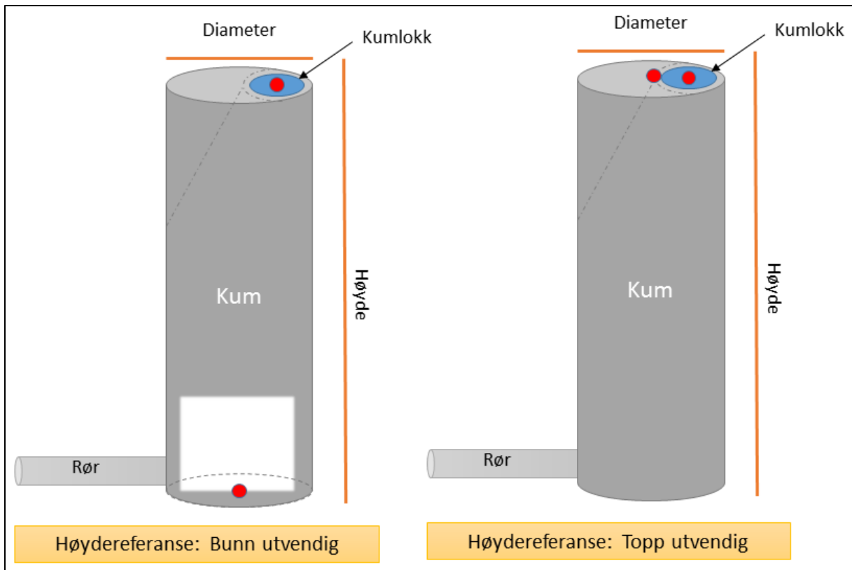
Figur 21: Alle sirkulære kplingsobjekt skal registreres med senterpunkt samt diameter og høyde. Z-verdi skal registreres på bunn utvendig kum, - dersom ikke registrering av topp utvendig kum er avtalt. Kplingsobjektets adkomst, her illustrert i form av kumlokk, skal stedfestes med senterpunkt for adkomsten.
