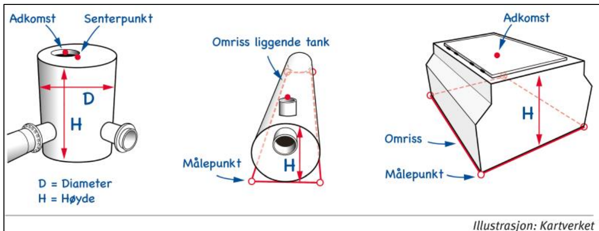
Figur 20: Eksempler på koplingsobjekt. Fra venstre: sirkulær i grunnriss, sirkulær i vertikalplanet, ikke sirkulære Illustrasjon: Kartverket
