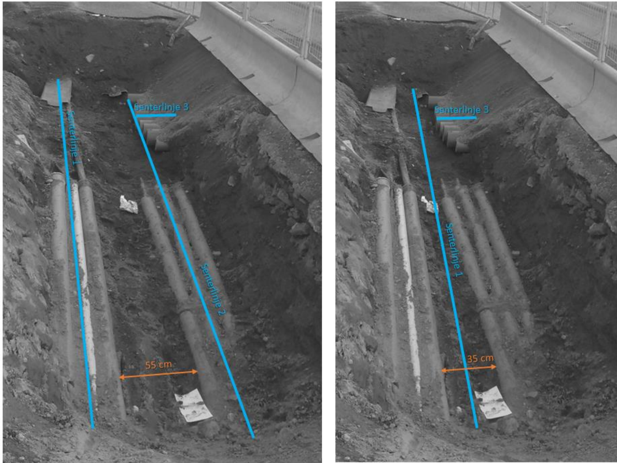
Figur 9: Dersom avstanden mellom to ledningsgrupper i grunnen er større enn 40 centimeter i grunnriss og/eller høyde, innenfor område type 1, skal hver av ledningsgruppene registreres med en senterlinje (ledningstrase). Dersom avstanden er under 40 centimeter er det opp til ledningseier å avgjøre om man ønsker å registrere en eller flere senterlinjer (ledningstraseer).
