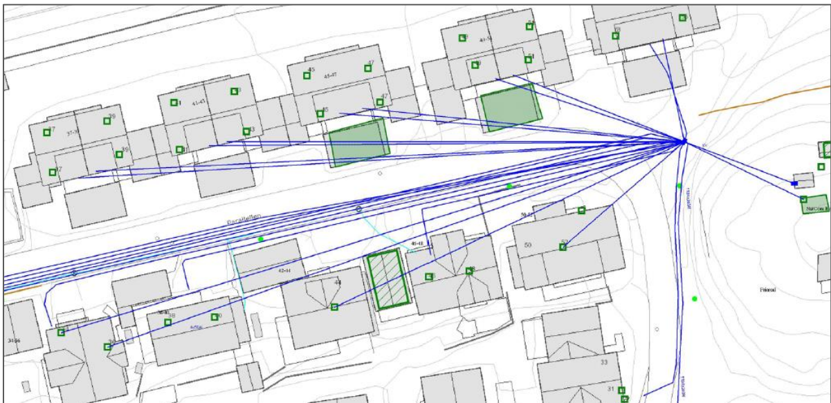
Figur 26: Eksempel på «Ledningskart» med rette linjer mellom koplingsobjekt og terminering hos abonnent. Her må det påvises hvor kablene går dersom det skal graves mellom husrekkene.
