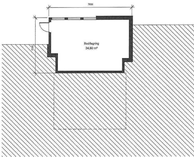
1 U. etasje 1 : 100
