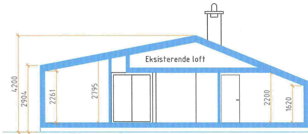
SNITT A-B (sett fra Øst)
