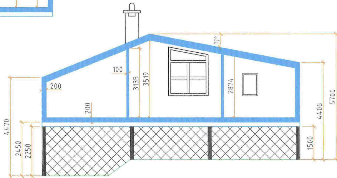
SNITT C-D (sett fra vest)
