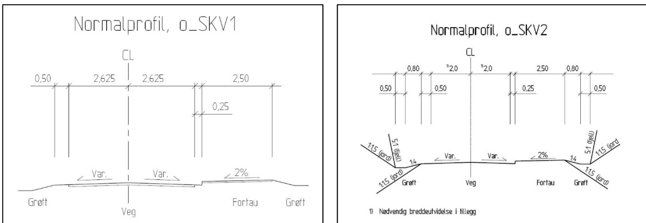
Figur 29. Normalprofil for vegane o_SKV1 og o_SKV2.
