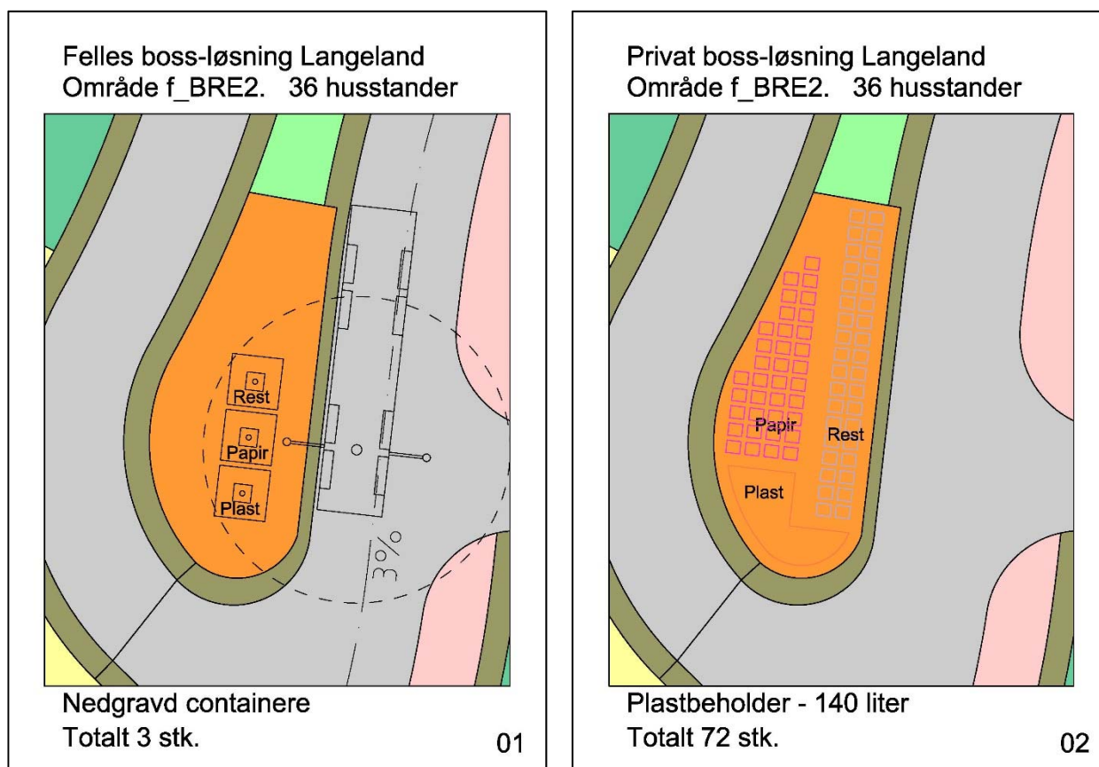
Figur 28. Bilda viser alternative løysingar for renovasjon. 1) Nedgrave løysing med container og 2) ordinær løysing med avfallsdunkar for restavfall og papir og plass for plastavfall.
