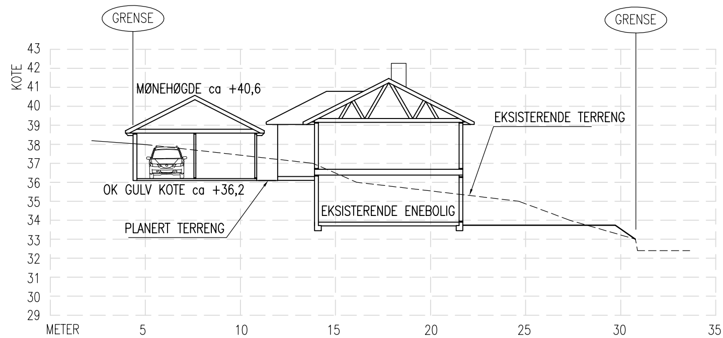
TERRENGPROFIL A-A
