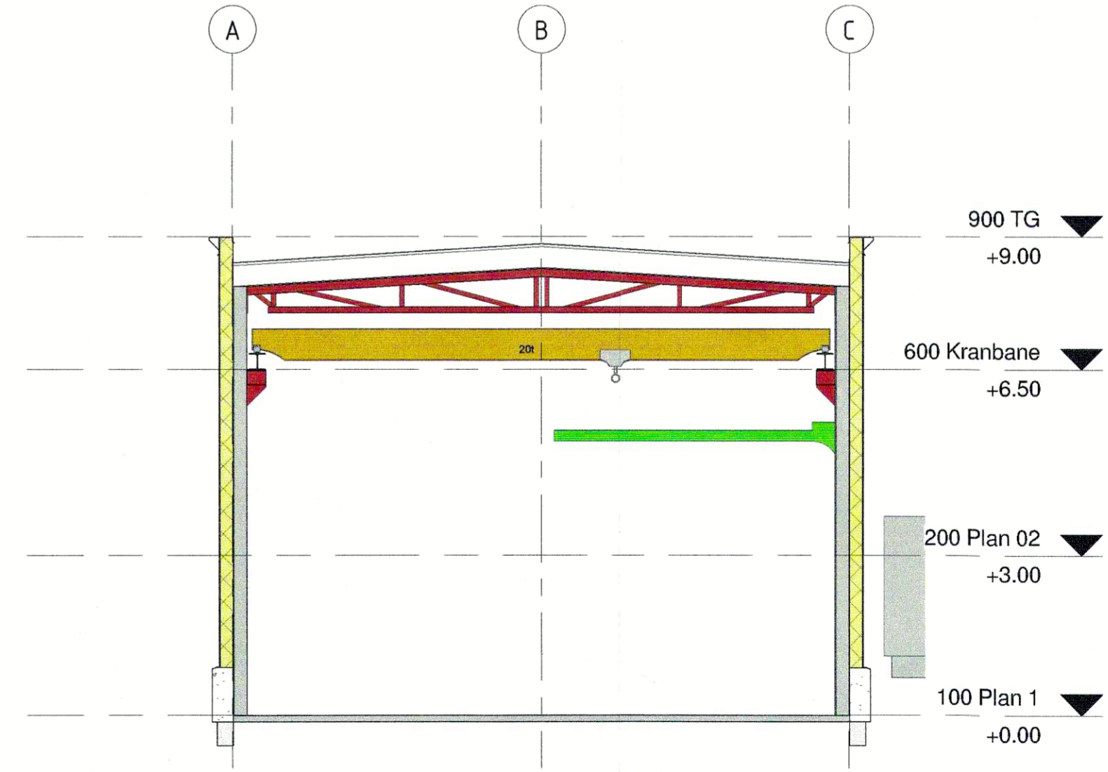
C-C 1 : 100
