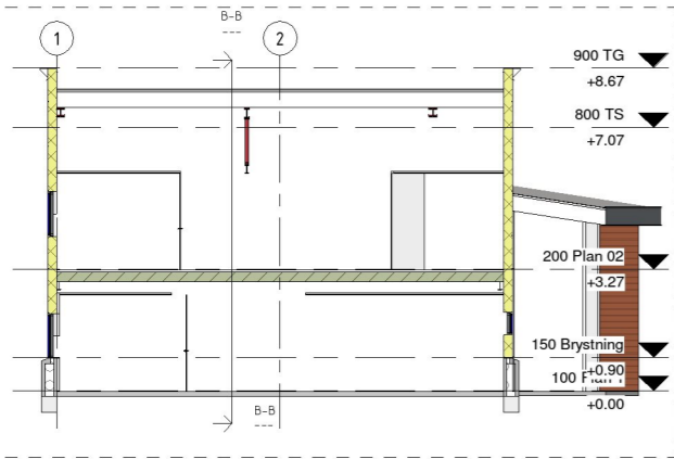
A-A 1:100
