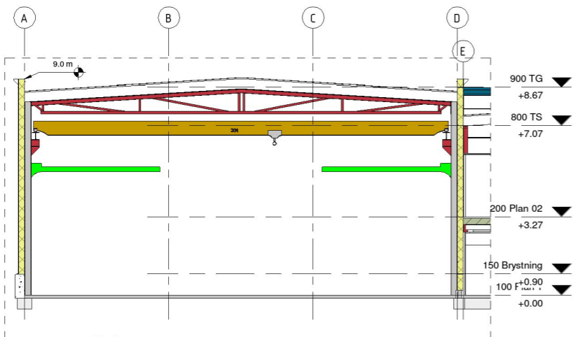
C-C 1:100
