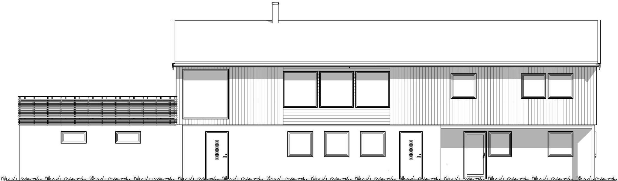
FASADE 1
