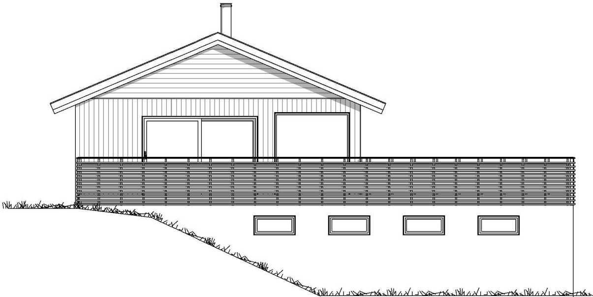
FASADE 4
