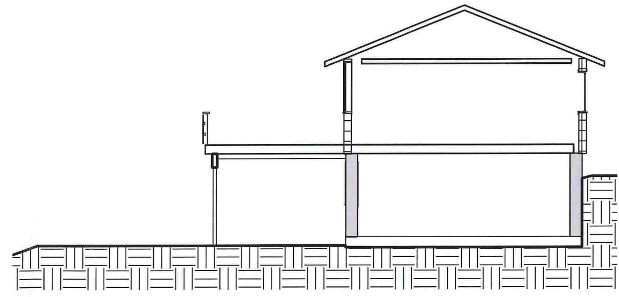
2 Snitt Øst 1 : 100
