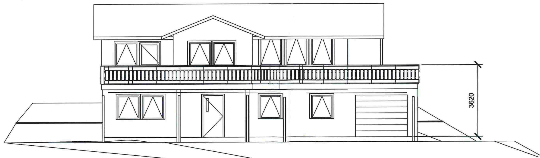
3 West 1 : 100
