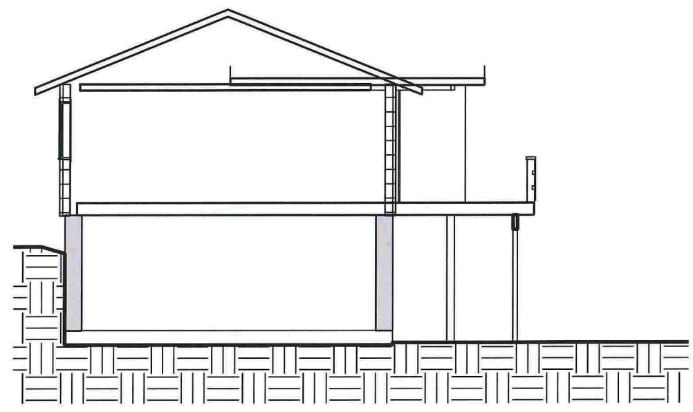
1 Snitt Vest 1 : 100
