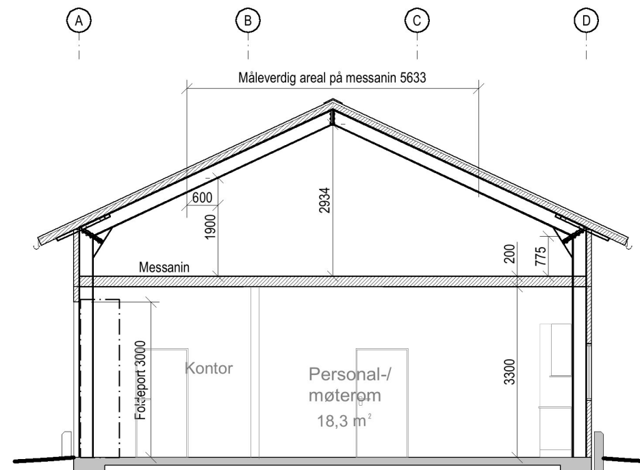
SNITT 2
