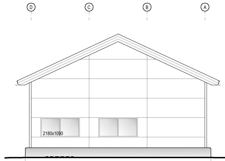
FASADE C
