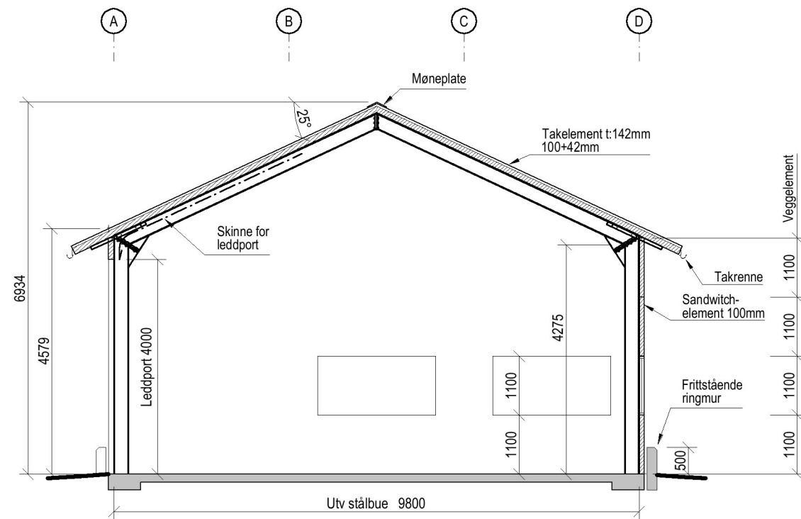
SNITT 1
