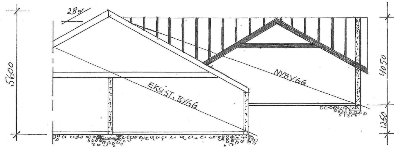
SNITT B-B
