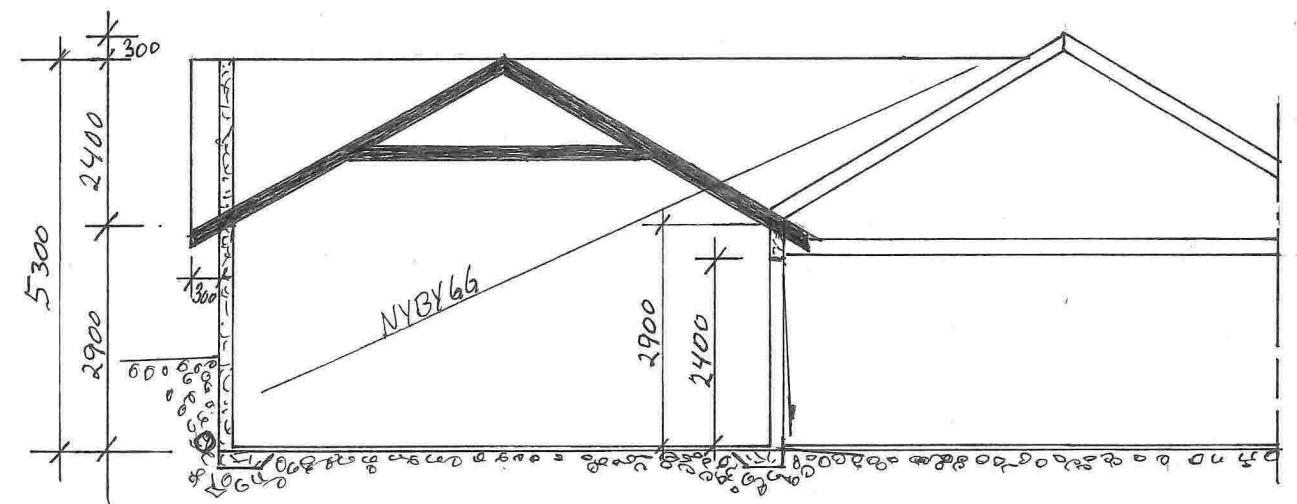
SNITT C-C
