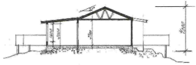
SNITT A-A
