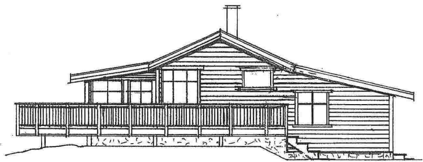
FASADE MOT ØST TILBYGG
