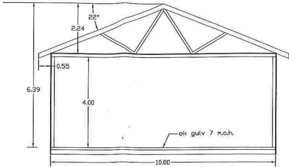
snitt A
