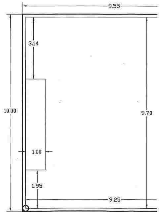
2. etasje
