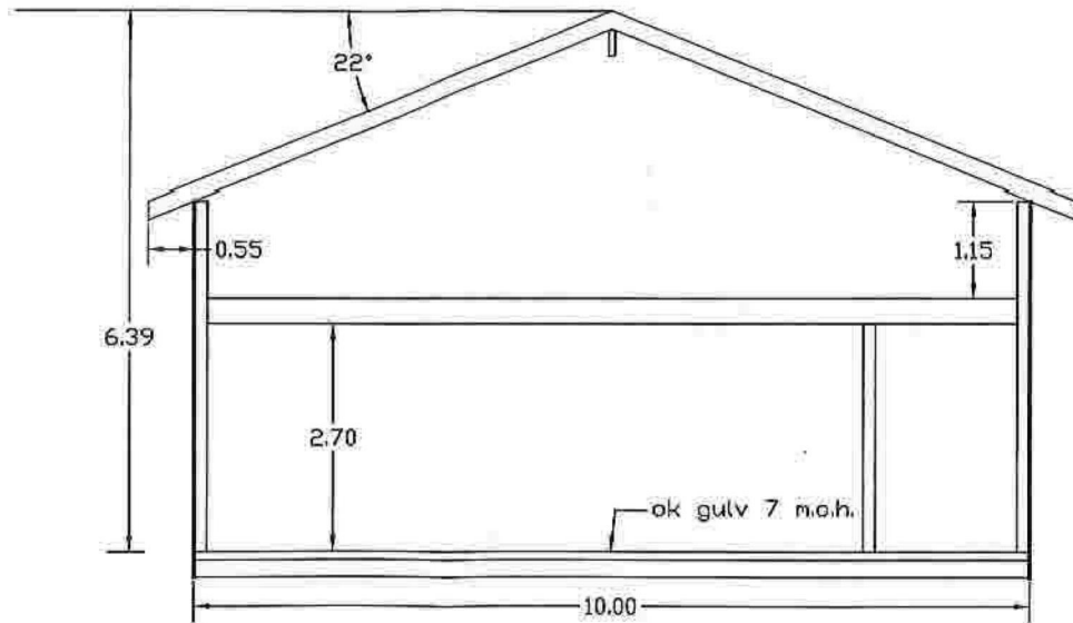
snitt B
