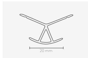
ALU PROFIL, 135° UTVENDIG HJØRNEPROFIL
