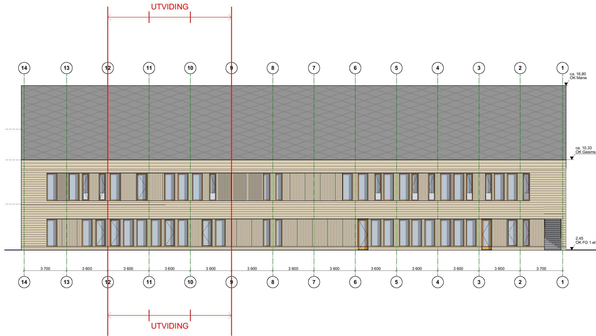
Fasade Nord
