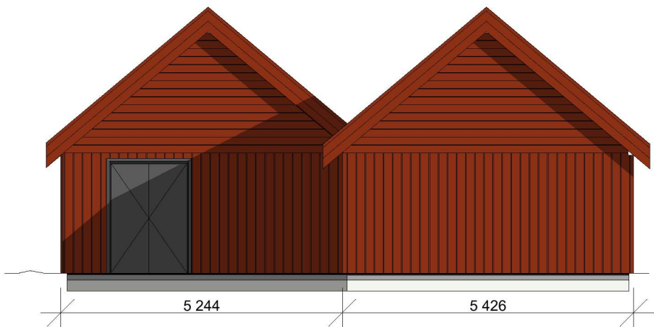
FASADE NORD
