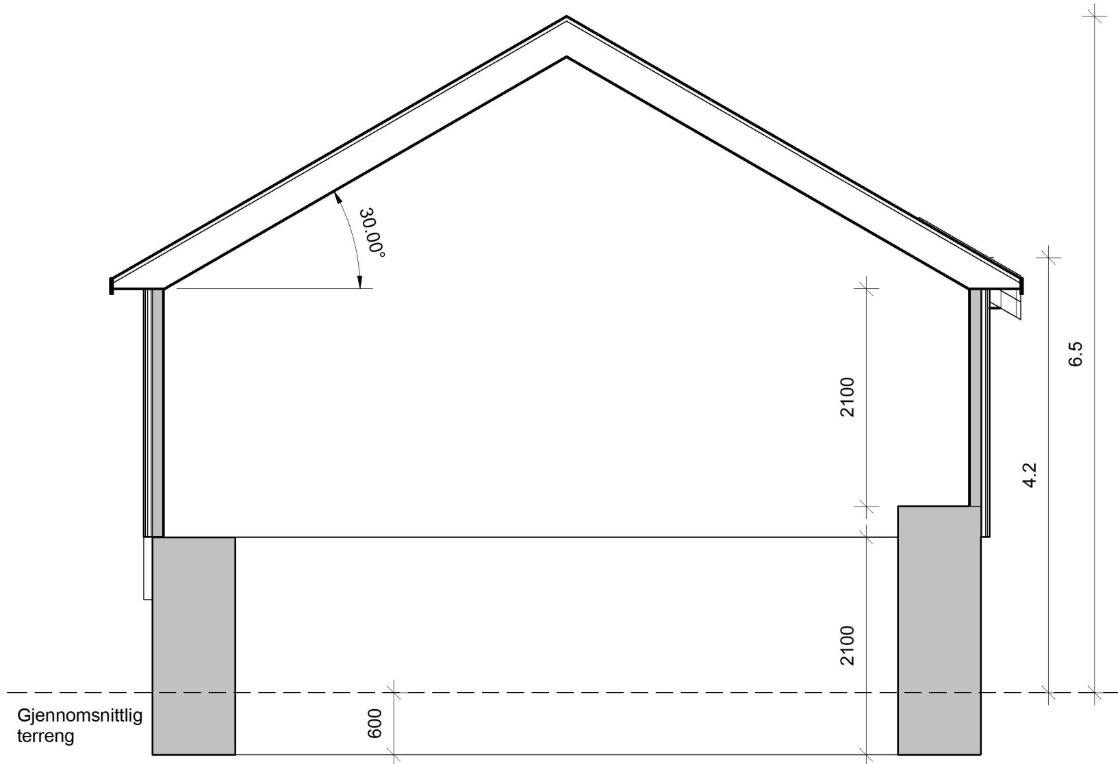
1 SNITT A-A 1 : 50
