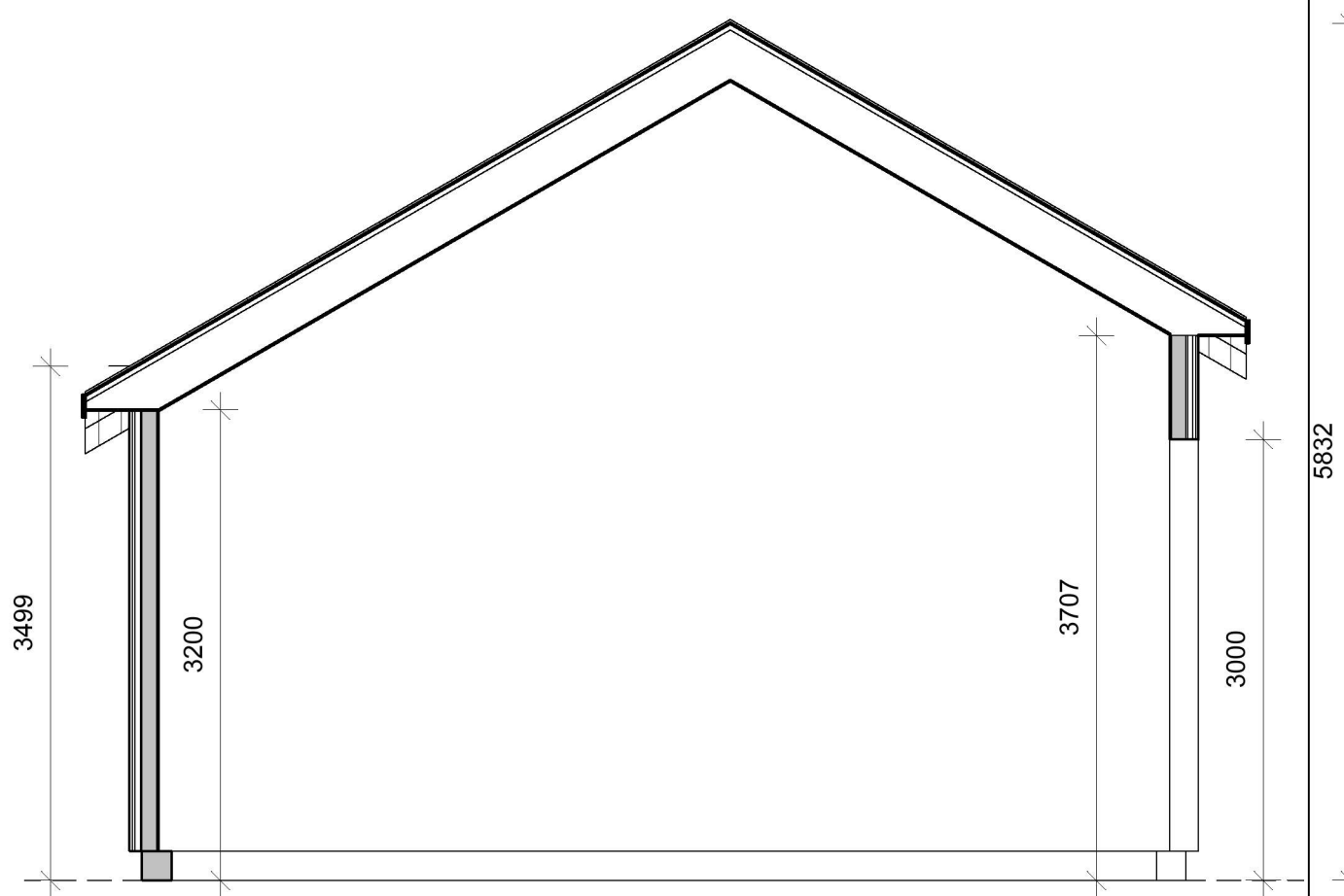
2 SNITT B-B 1 : 50
