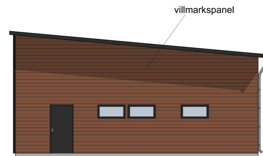
1:100 Fasade Sør
