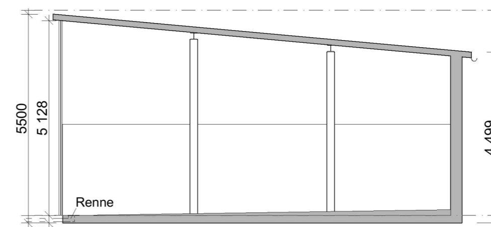
1:100 Snitt A
