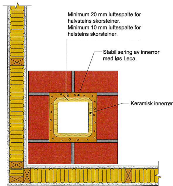
Leca Rehabiliteringssytem (luftet løsning) i teglskorstein. Stabilisering av innerrør med løs Leca.
