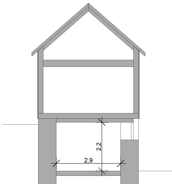
SNITT A-A
