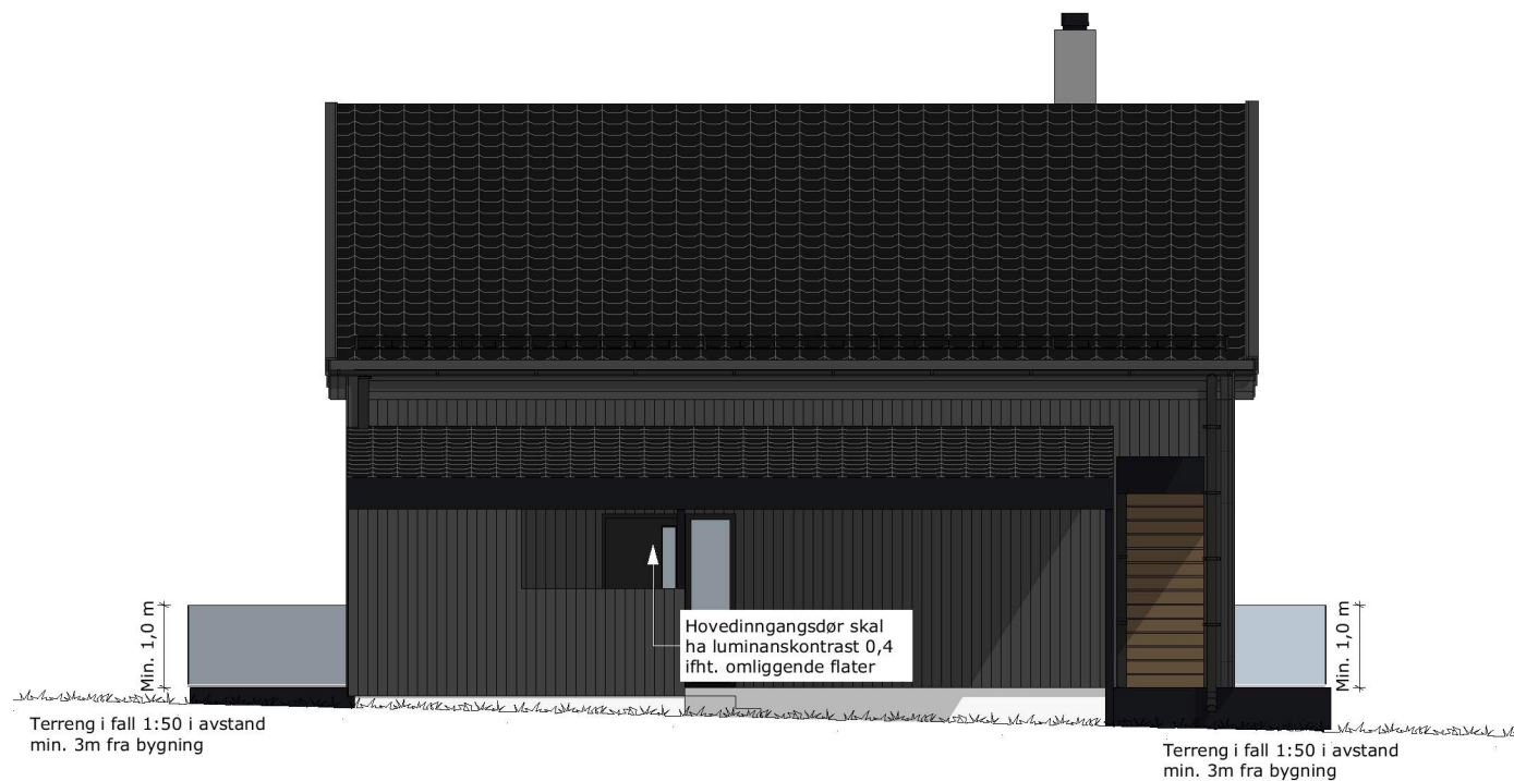
Fasade Øst
