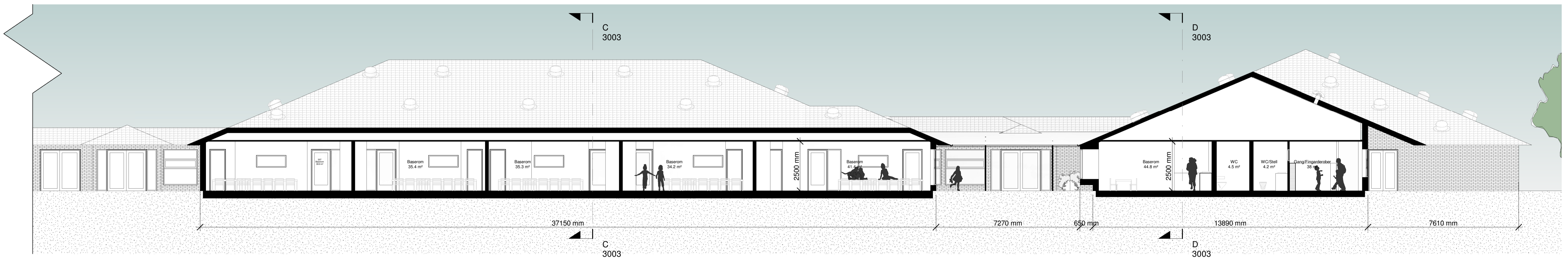
Snitt A 1 : 100
