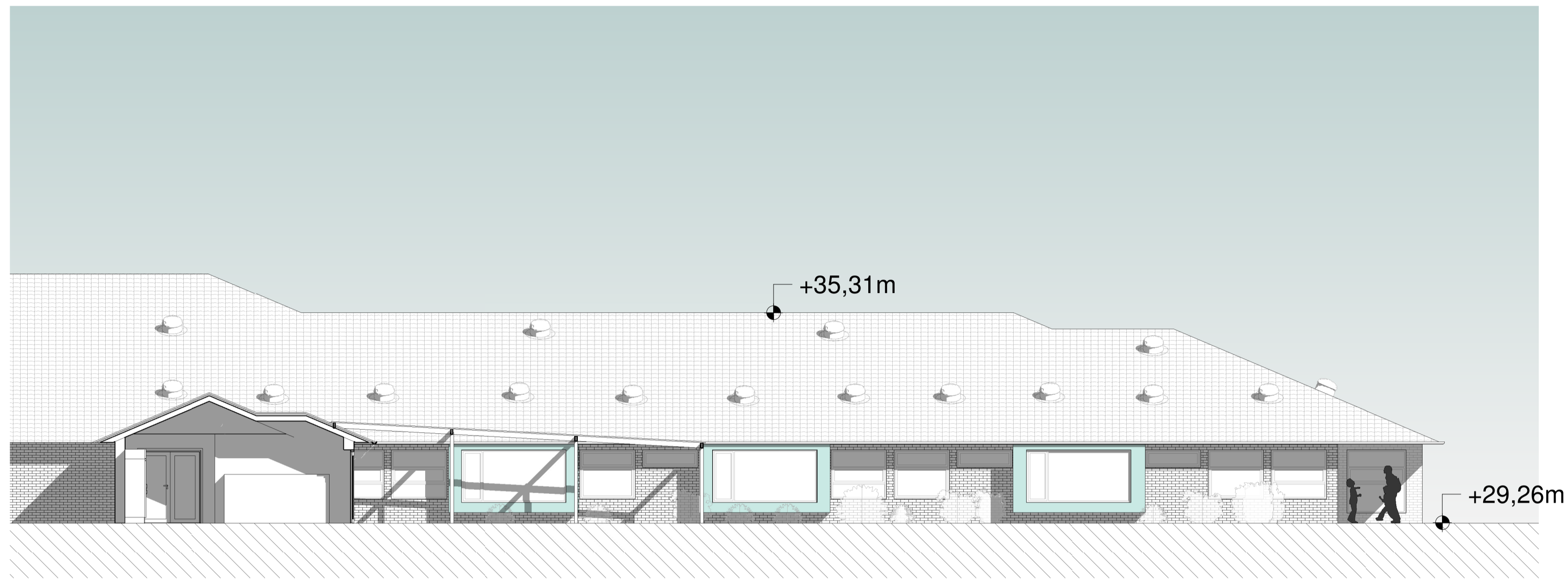
Fasade ØST 1 : 100
