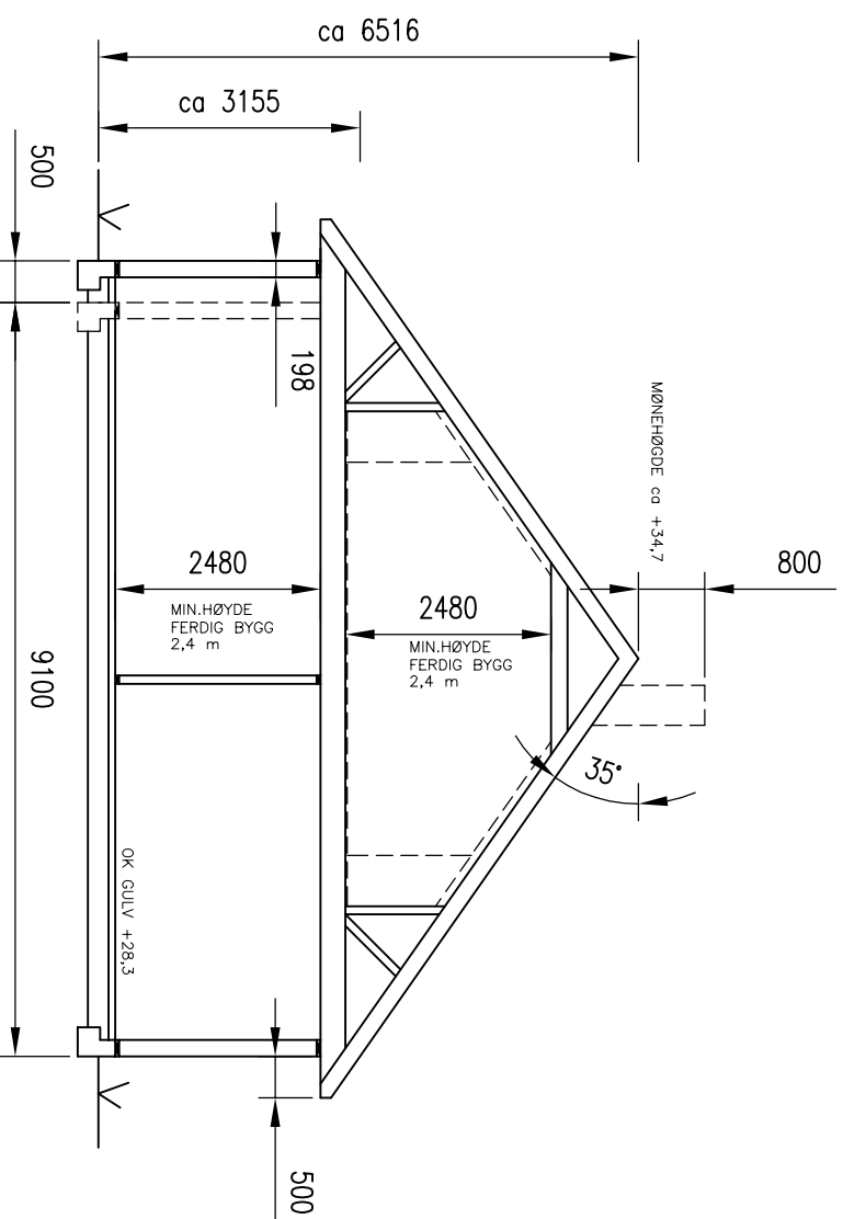
TYPISK SNITT
