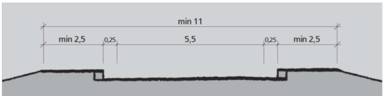
Figur 12. Normalprofil Fv. 409
