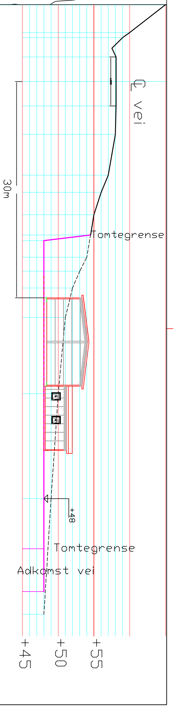
Tverrsnitt - terrengsnitt fra vei
