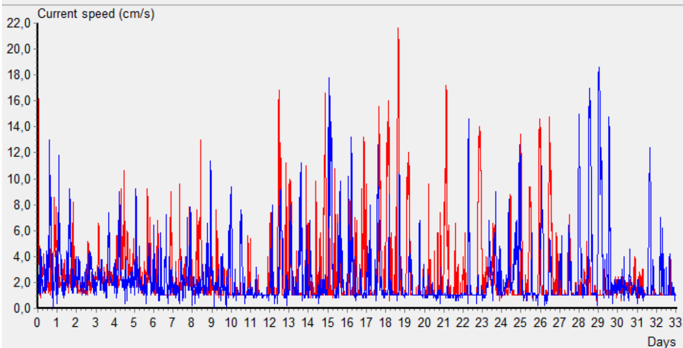
Figur 8.11 Figuren viser tidsdiagram for strømsstyrken uavhengig av retning. Blå kurve gjelder for 15 m og rød for 5 m.
