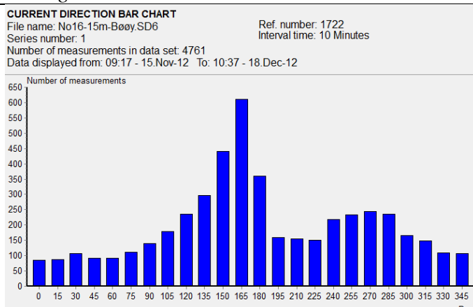
Figur 8.6 Oversikt over fordeling i de ulike hastighetene og fordeling i de ulike retningene i måleperioden samt maksimal strøm i de ulike retningene.
