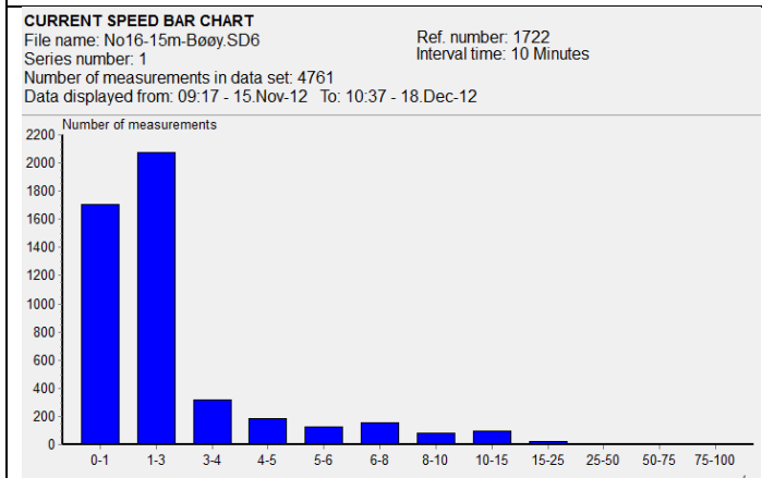
Figur 8.7 Antall målinger i de ulike hastighetene.
