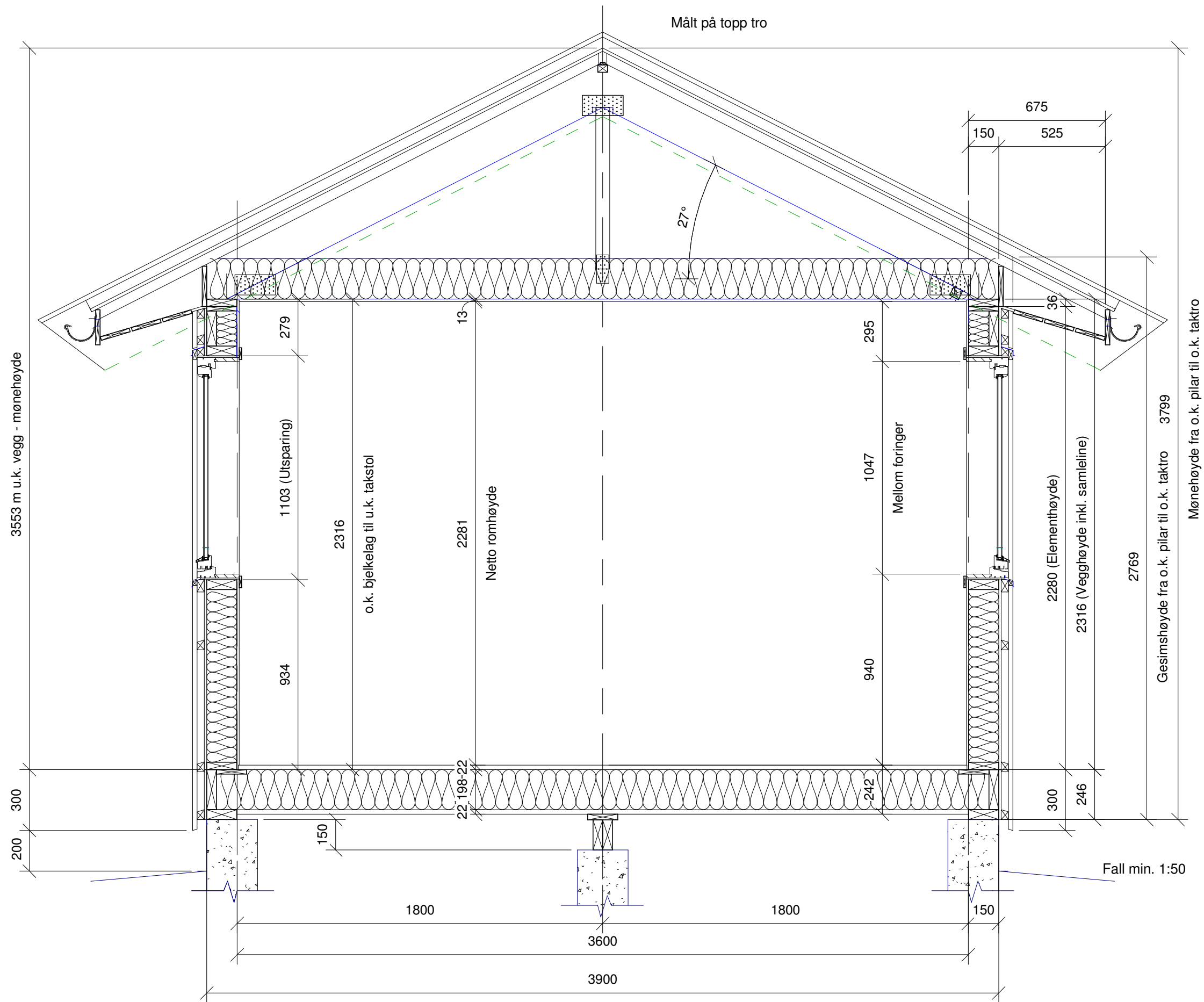
Anneks 2016 - 27gr M3600 m. takstol Snitt anneks med bjelkelag 30.08.16 RW
