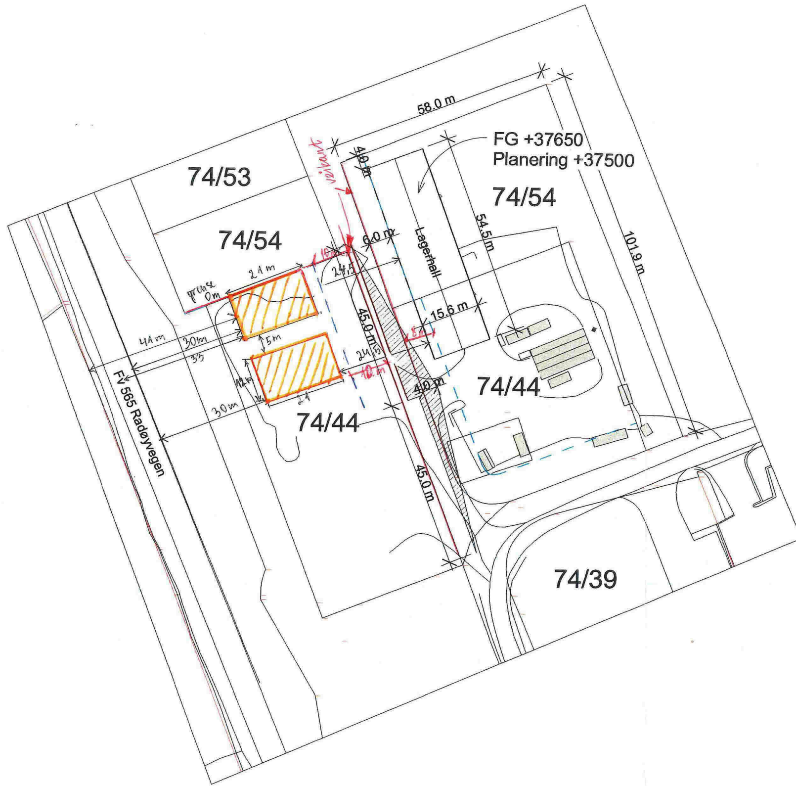
Situasjonsplan 1 : 1000
