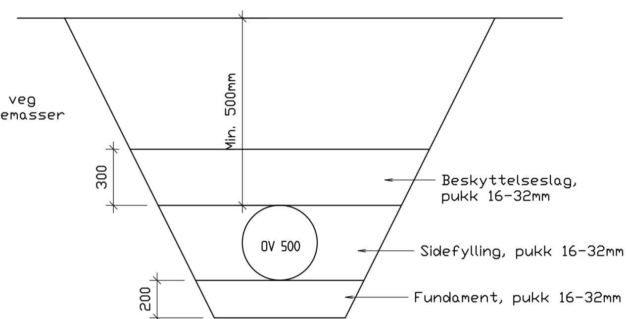
GRØFTESNITT 1. M=1:20 Ø500mm betong overvannsledning
