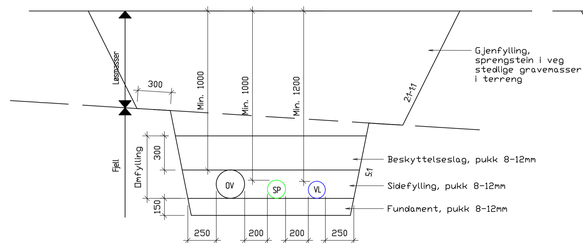
TYPISK GRØFTESNITT. M=1:20 Vann-, spillvann- og overvannsledning
