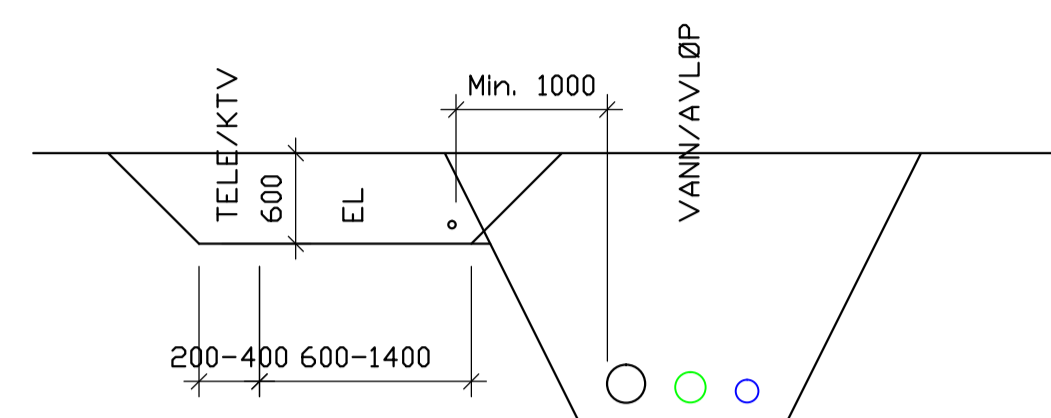
GRØFTESNITT 2. M=1:50 Tele/KTV, strøm og vann/avløp
