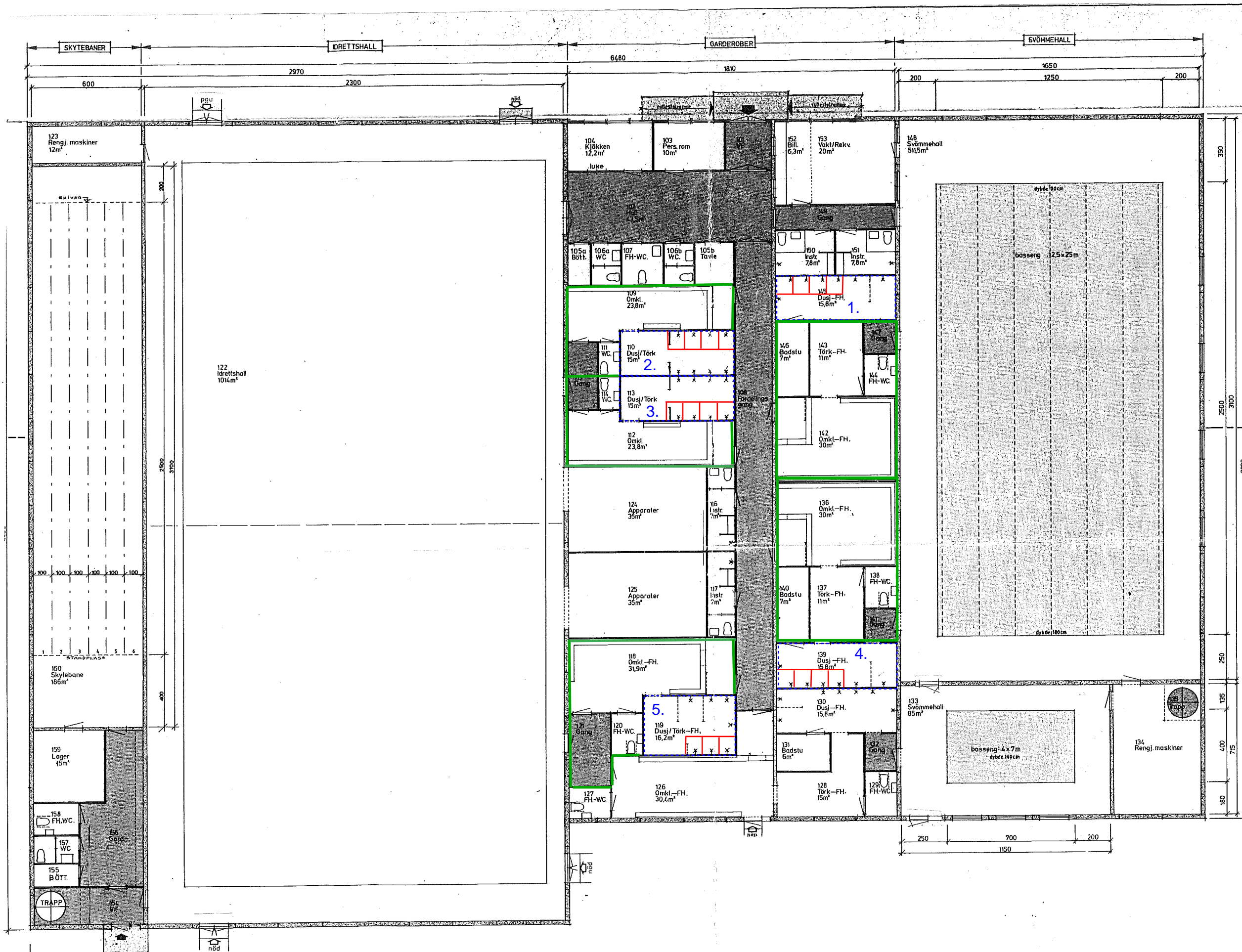
PLAN-1. ETASJE Brutto areal : 2687m 2
