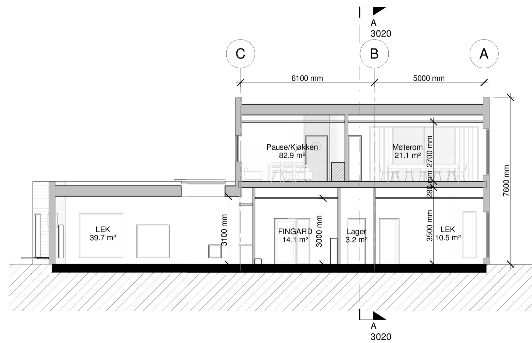
Snitt CC 1 : 100
