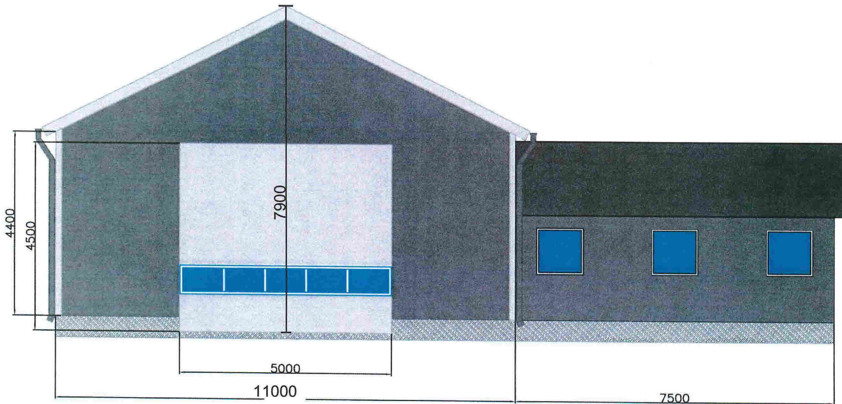
FASADE 2
