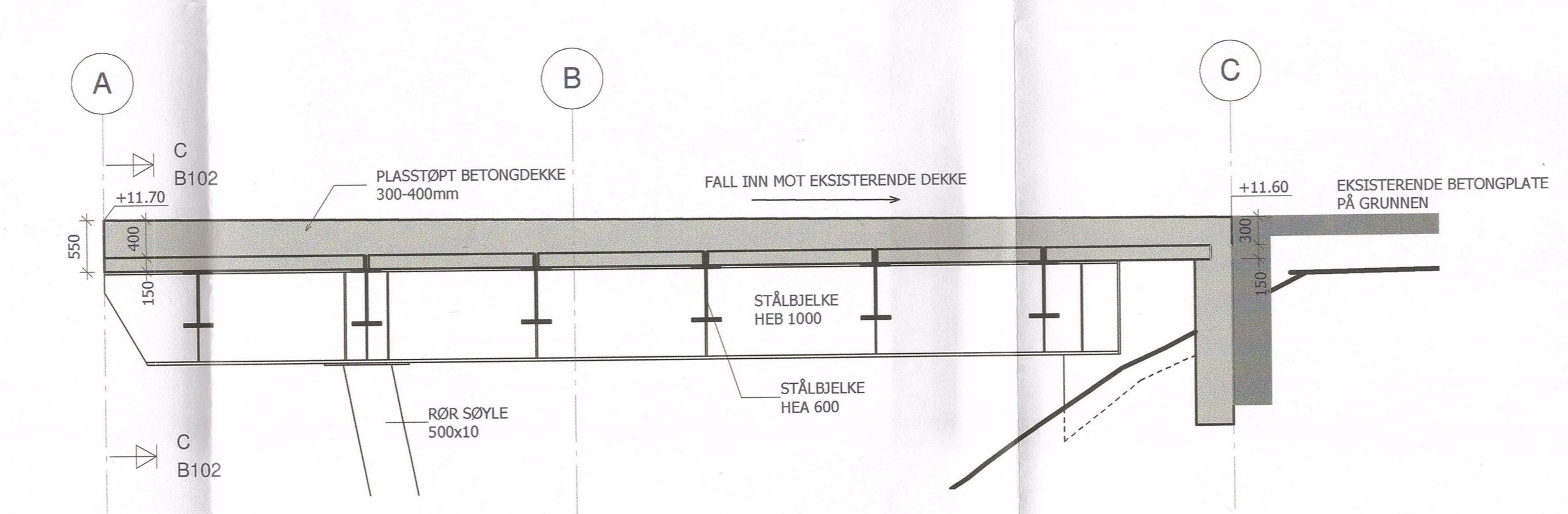
SNITT E 1 : 50
