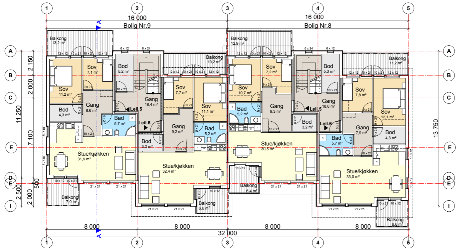
Plan 2 etasje
