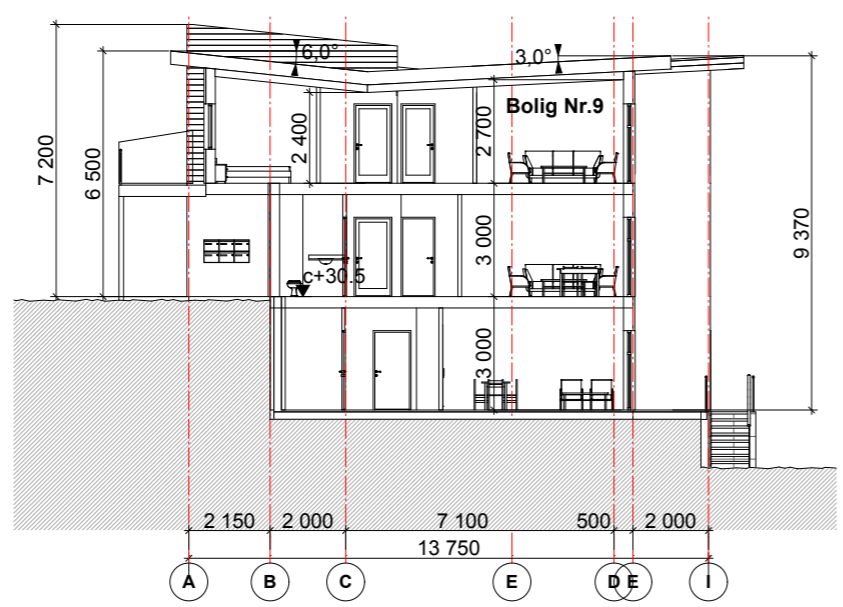
Snitt A-A
