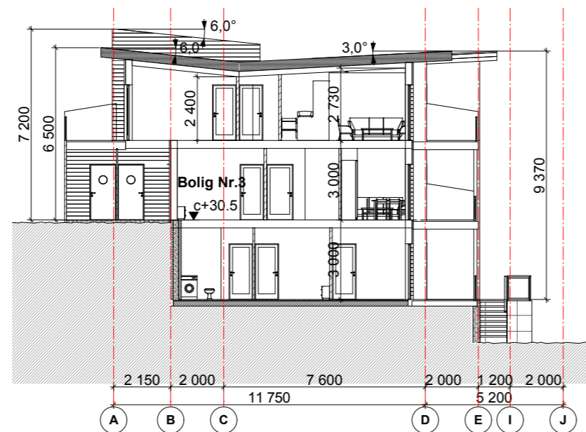
Snitt A-A
