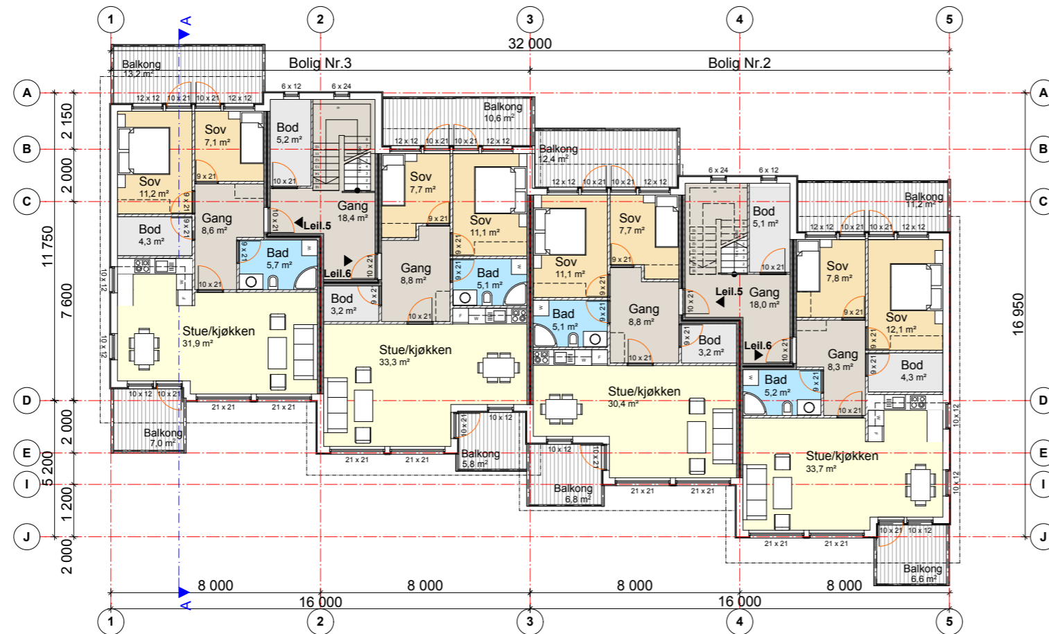
Plan 2 etasje
