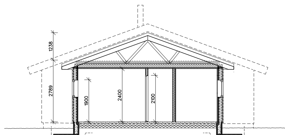
SNITT C-C
