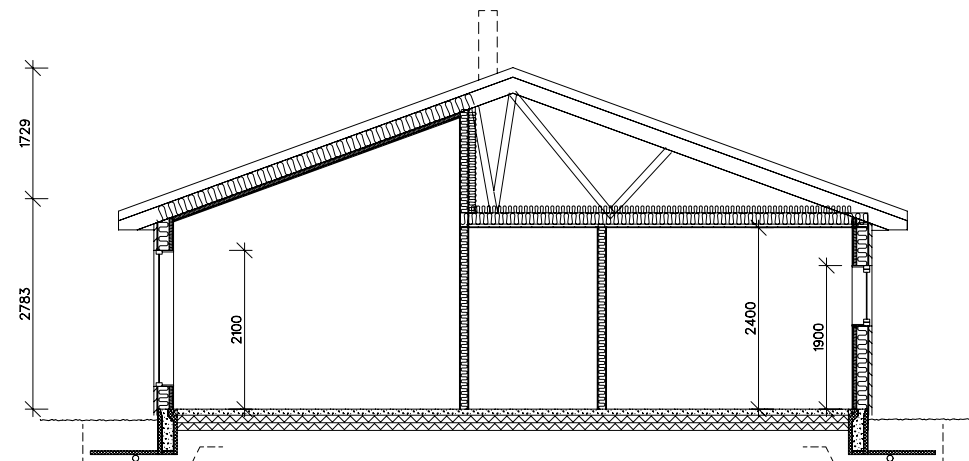
SNITT B-B
