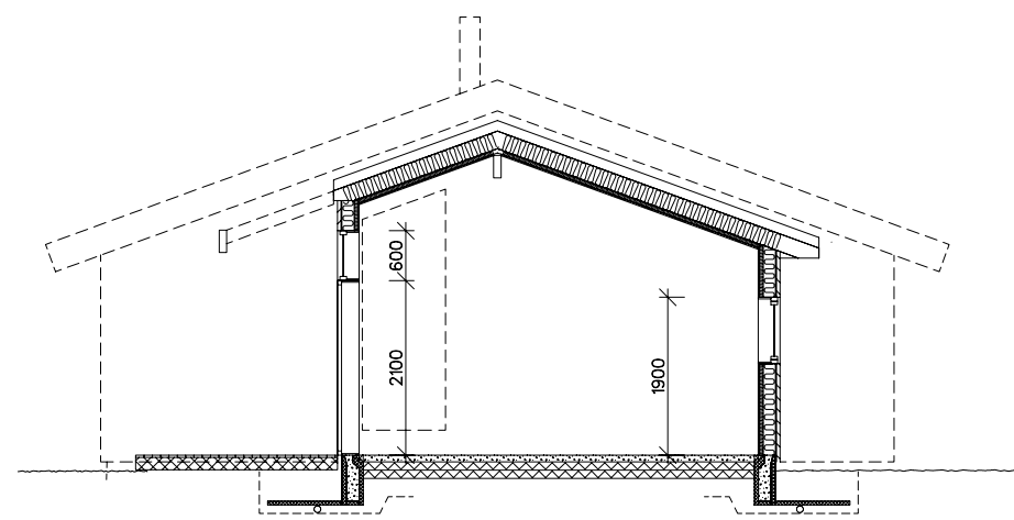
SNITT A-A
