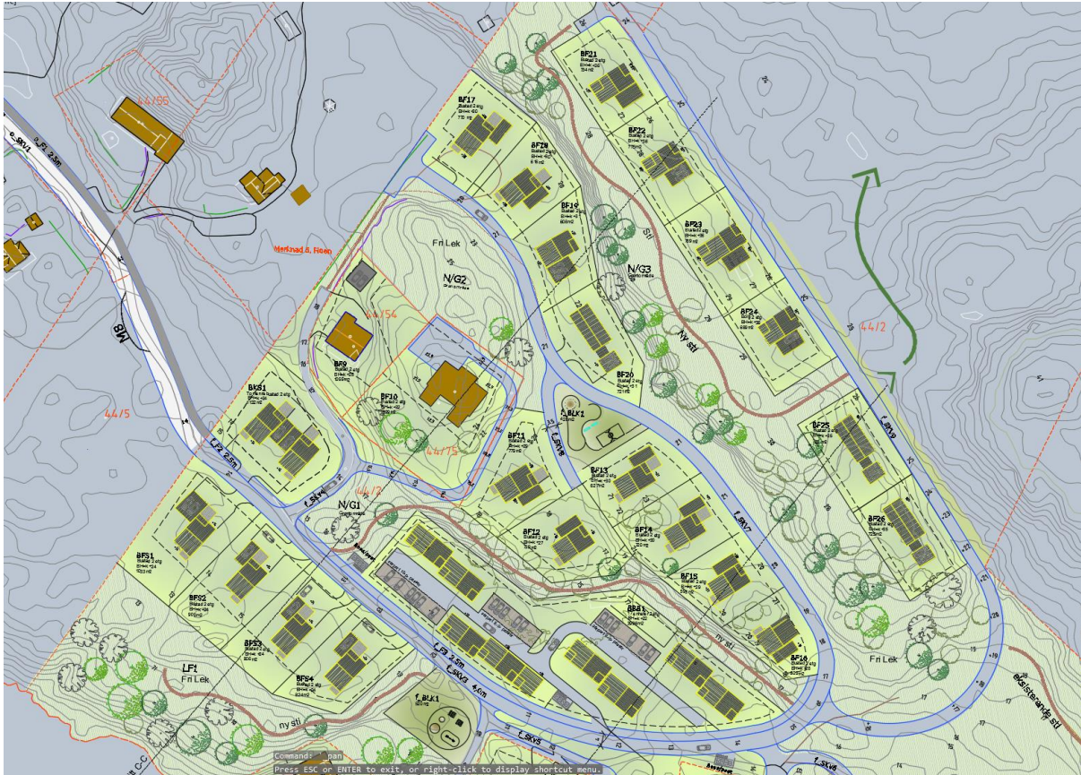
Utsnitt illustrasjonsplan BFS.
