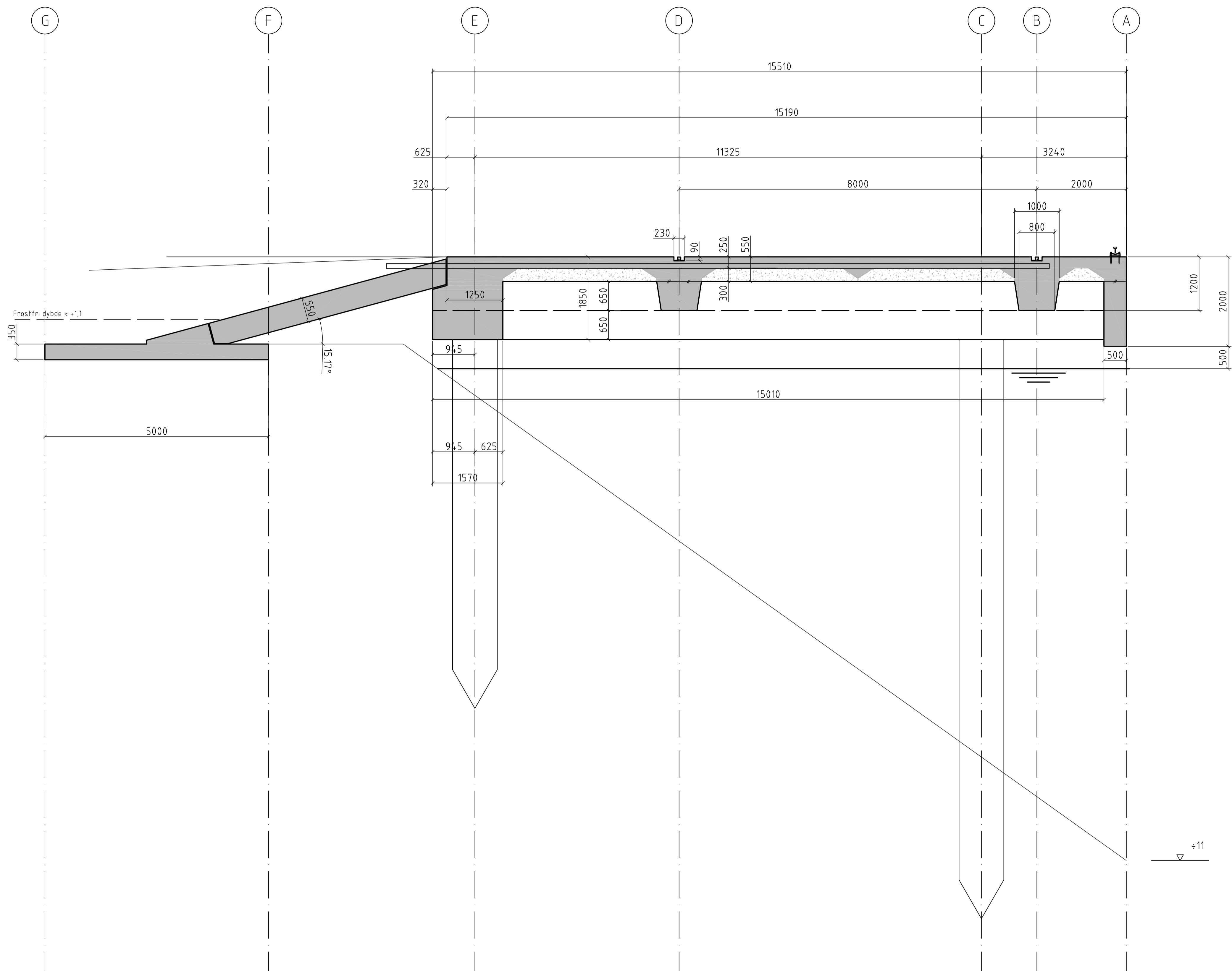
SNITT 1-1 TYPISK SNITT KAI 1:50
