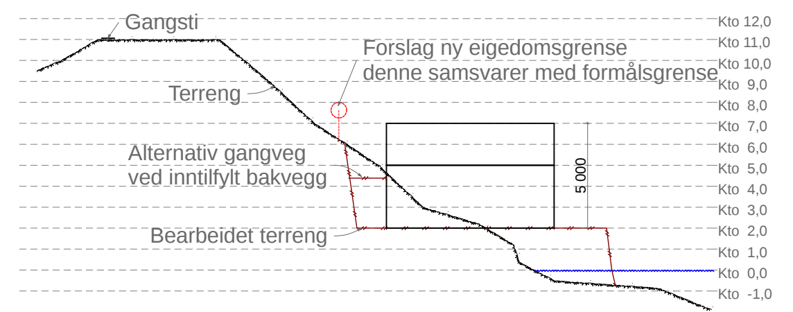
PRINSIPPSKISSE TERRENGPROFIL OG PLASSERING NAUST MED KAI
