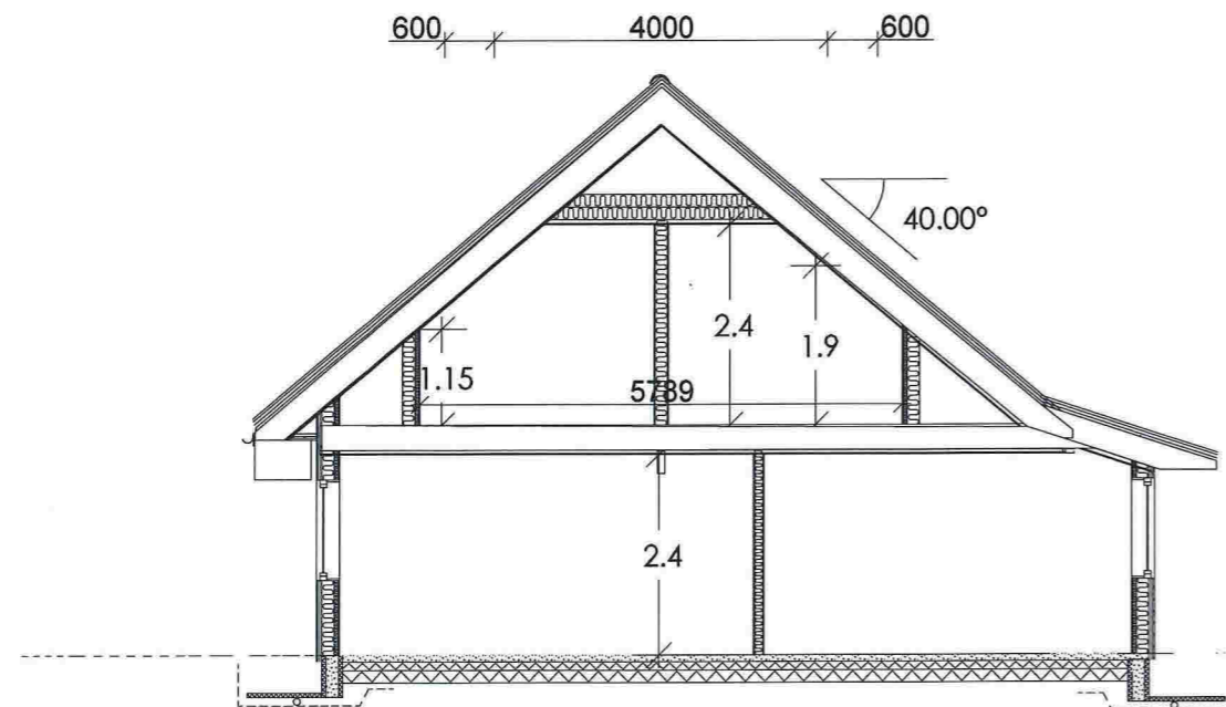
SNITT B-B
