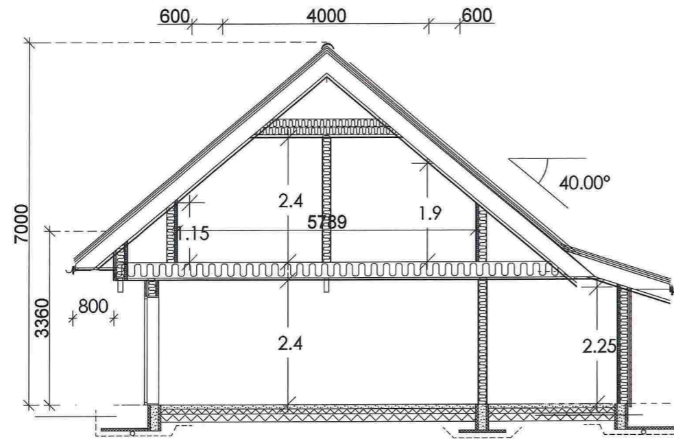
SNITT A-A
