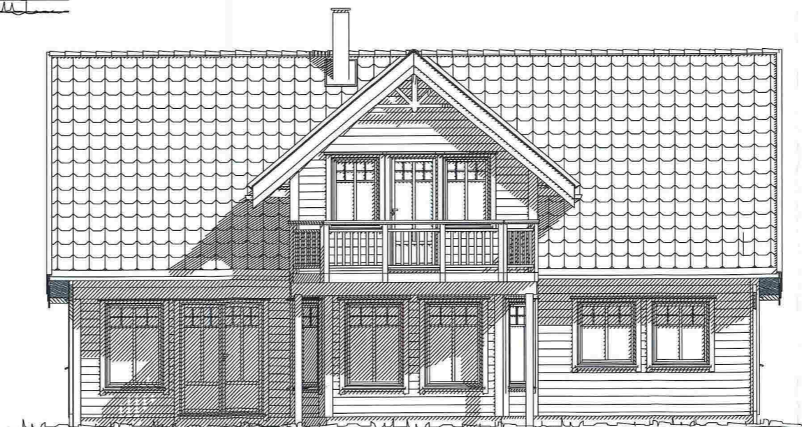
FASADE SØR
