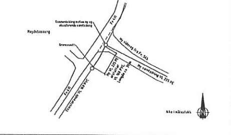
Skisse / Grensesnitt for sammenkobling mellom ny og eksisterende vannledning ved Haukåsen
