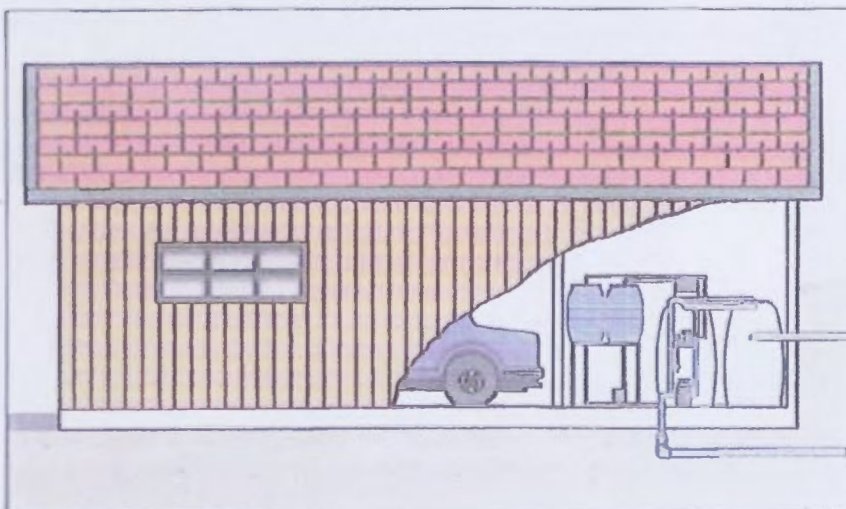
Anlegg for en hus- eller hytteenhet plassert på gulv i garasje
