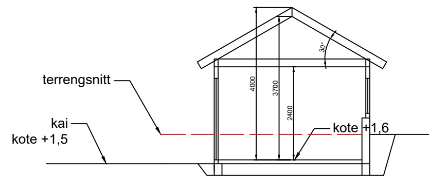
Snitt A-A
