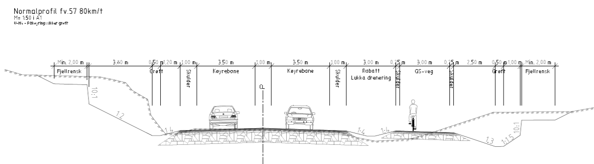
Figur 2 Normalprofil for ny fv. 57 med gang- og sykkelveg og sone 80 km/t. Kjelde: Multiconsult / SVV.
