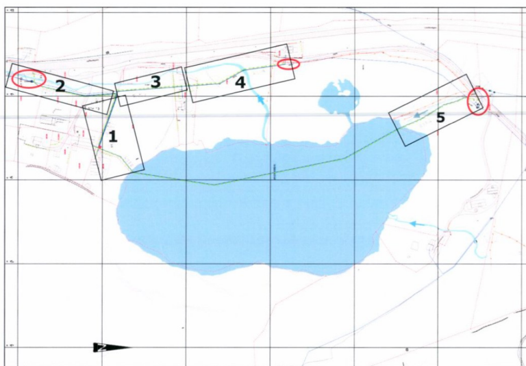
Fig. 6. Traséer for prosjekterte VA-ledningsnett (grønne linjer). 3 endepunkter i prosjektert anlegg er vist med røde sirkler. Prosjekterte traséer er delt opp i 5 avsnitt, for mer detaljert omtale i rapporten. To innløpsbekker i nord, samt utløpselven fra midt på Isdalsvatnet, er markert. Kart: Haugen VVA AS.
