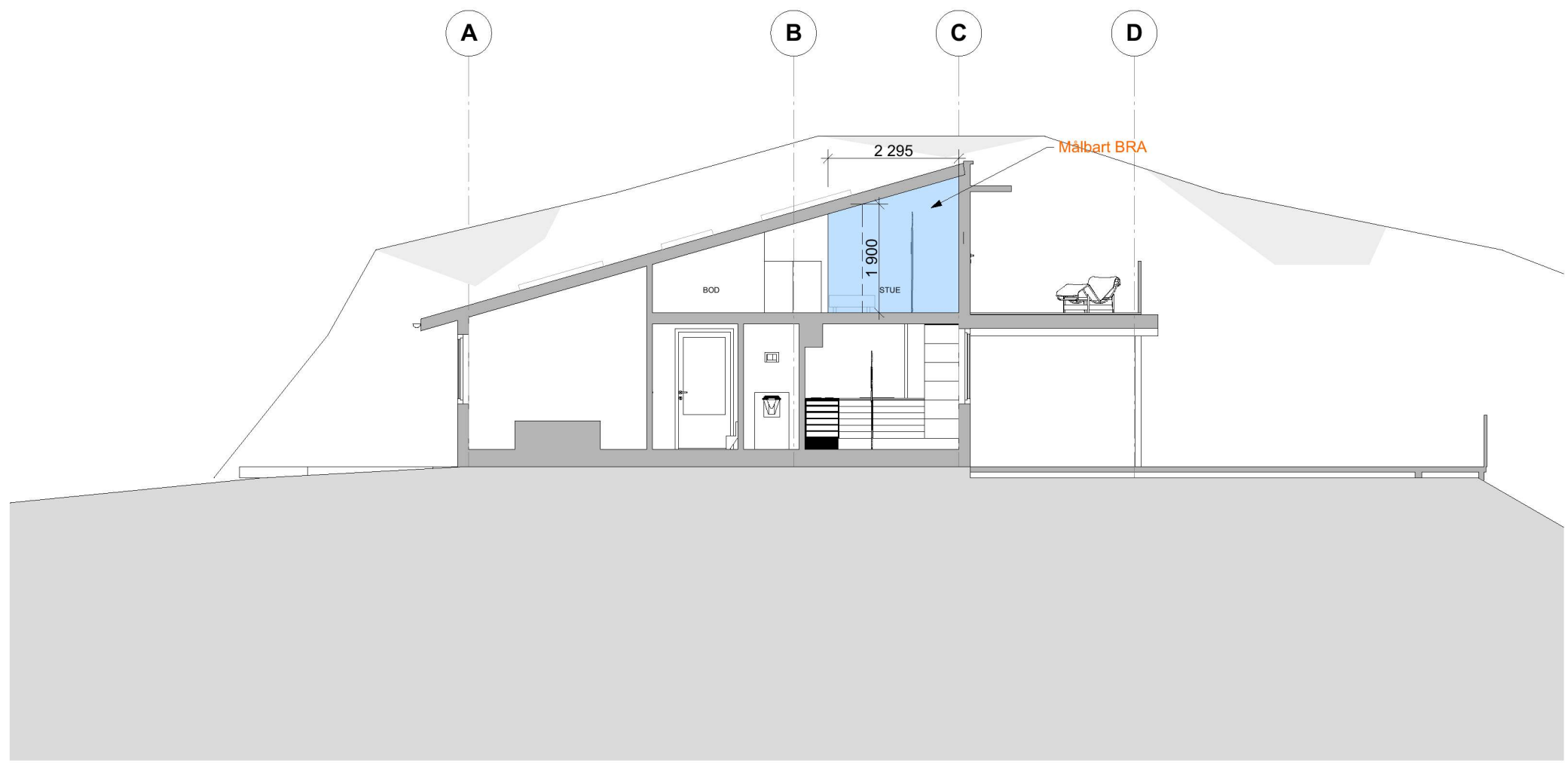
Snitt 5
